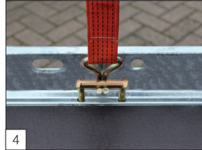
4 Serienausstattung: TÜV-geprüfte Verzurrbügel, integriert im Seitenrahmen: 1000 daN das Stück.
