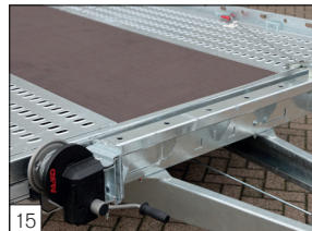
15 Option: Seilwinde 6-fach quer verstellbar statt normale Seilwinde.
