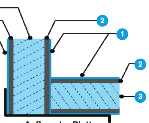
Aufbau der Platten 40 mm stark
